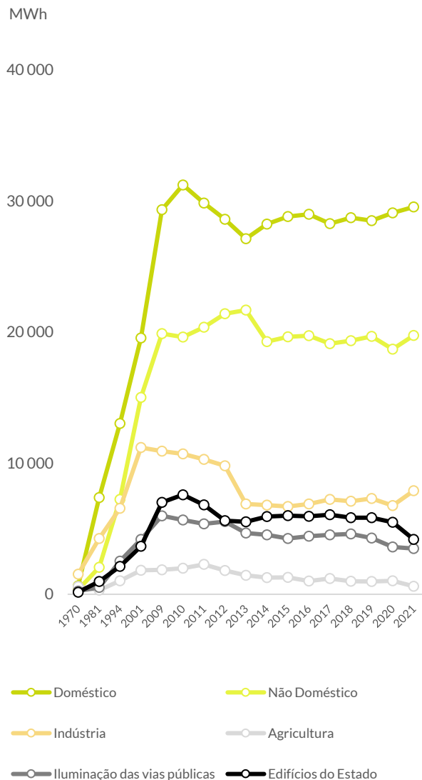
Gráfico 30 | Evolução do consumo de energia elétrica por tipo de consumo em Mirandela, 1970-2021
