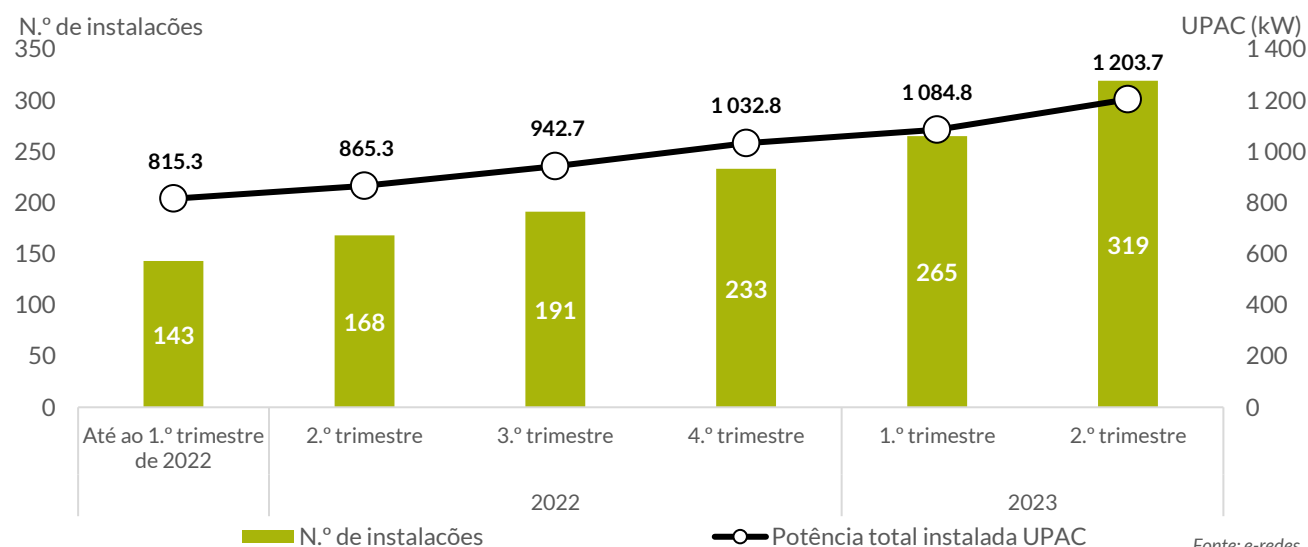
Gráfico 38 | Número de instalações e potência instalada de UPAC, em Mirandela, até ao 2.º trimestre de 2023
