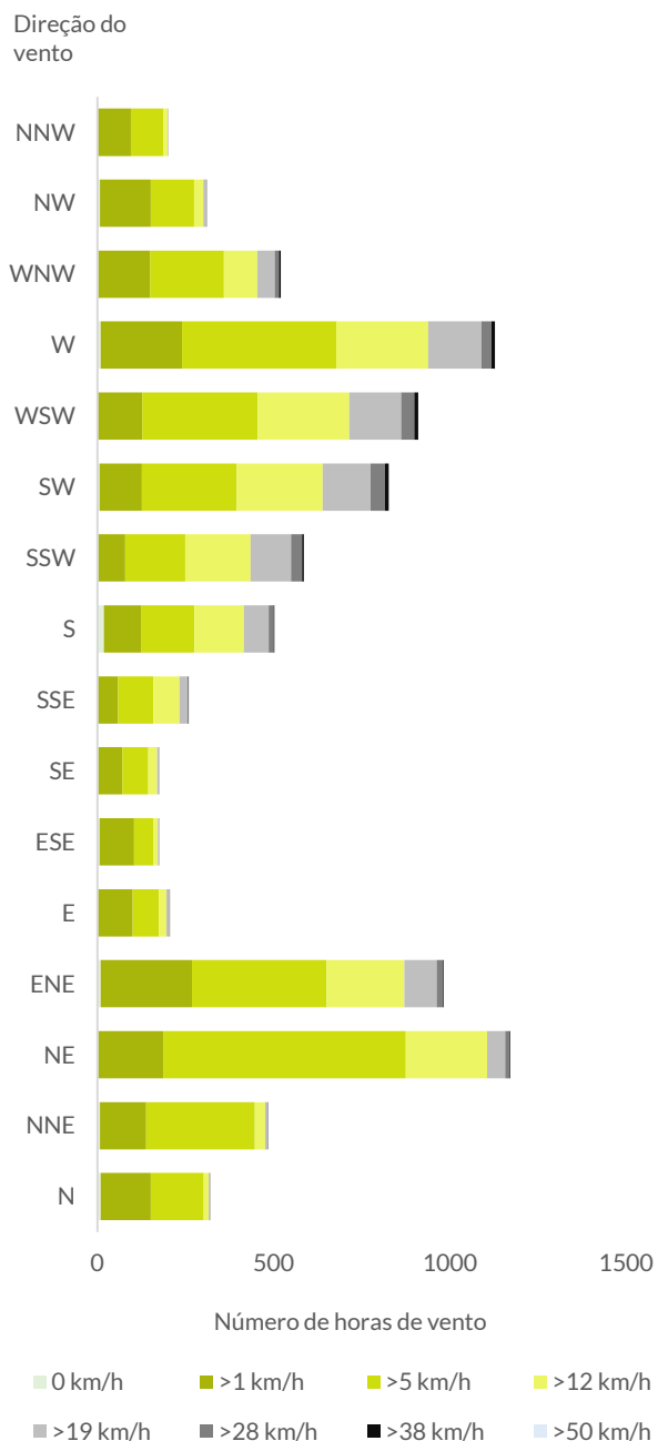
Gráfico 10 | Número de horas de vento por ano, velocidade e direção em Mirandela, média dos últimos 30 anos
