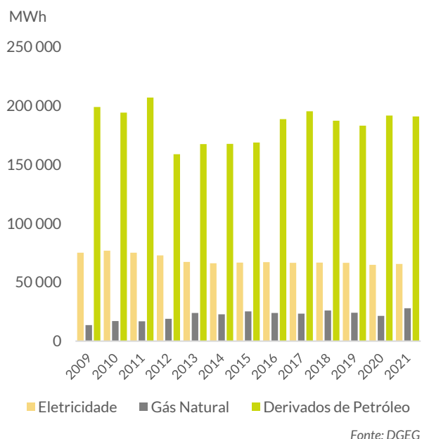
Gráfico 27 | Evolução do consumo de energia por tipo de vetor em Mirandela, 2009-2021
