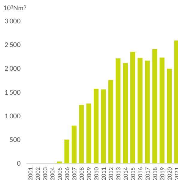
Gráfico 32 | Evolução do consumo de gás natural em Mirandela, 2001-2021
