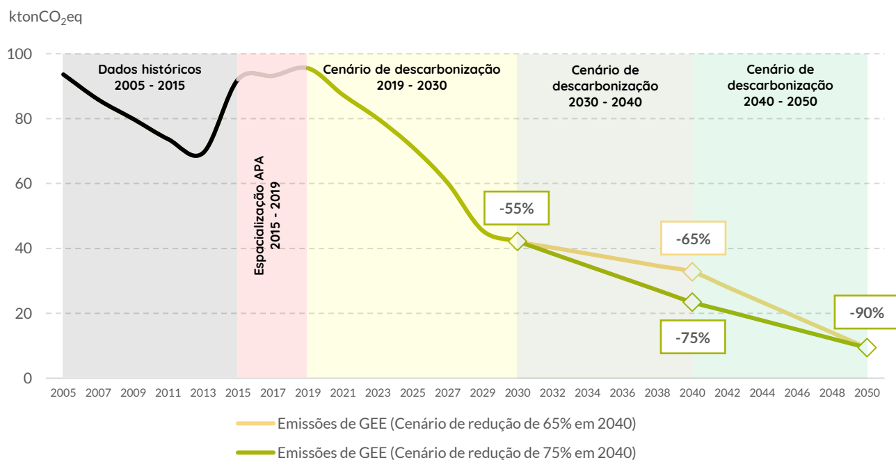
Gráfico 43 | Cenário de emissões de GEE 2030 – 2050, em Mirandela
