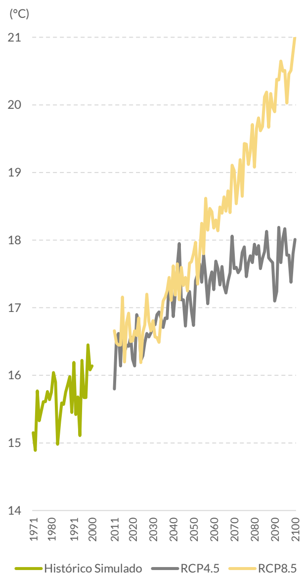
Gráfico 13 | Histórico simulado e anomalias da temperatura média máxima (°C) na região da CIM TTM
